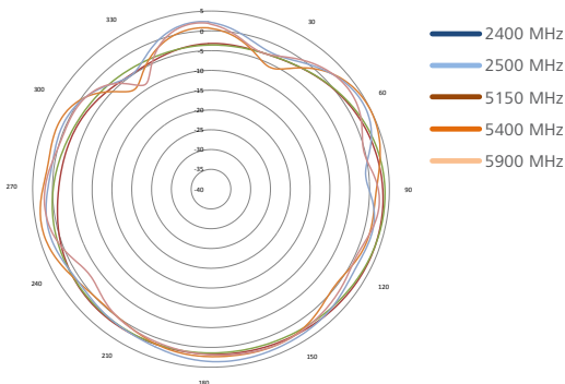
2.4 & 5 GHz h-plane
