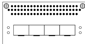
↓ LANCOM UF Extension Module 4× 1G SFP (UF-X60)
